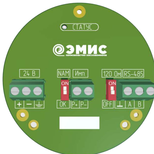
Рисунок 4.1. Плата клемм
