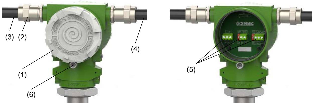
Рисунок 5.1. Электрическое подключение электронного блока
