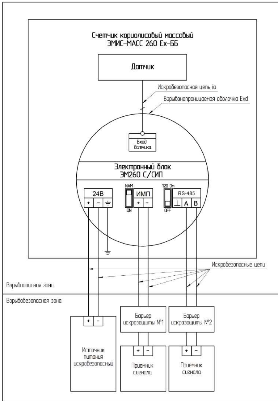
Рисунок 5.3. Электрическое подключение электронного блока исполнения Ех-ББ
